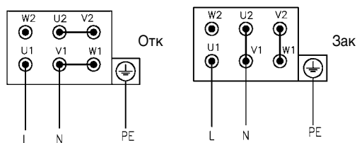
1-фазный двигатель
